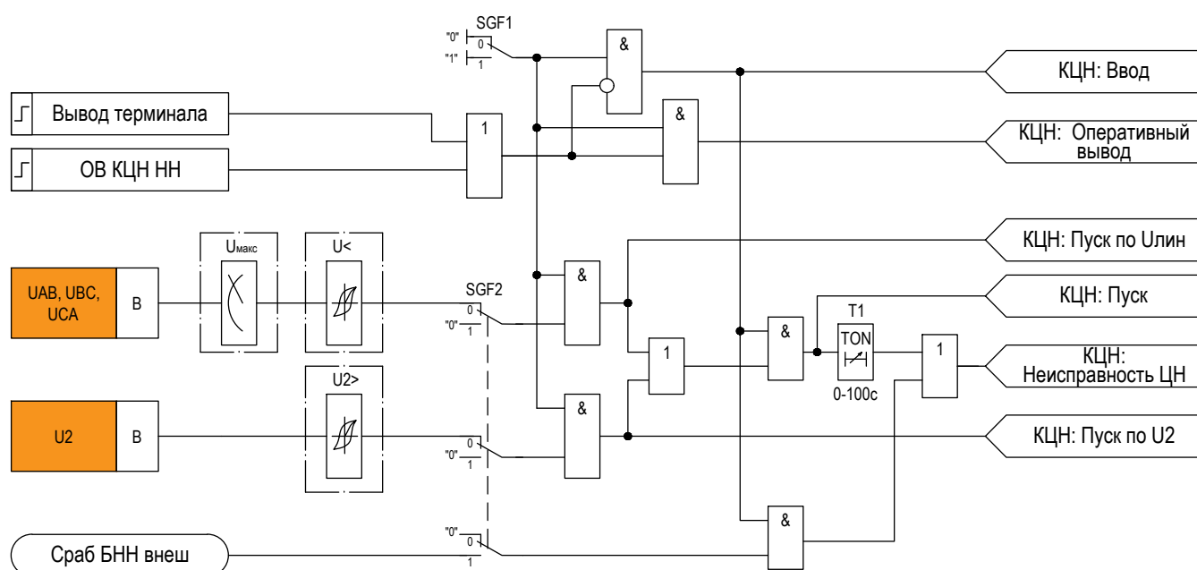
Рисунок 2.11 – Функциональная схема логики КЦН НН
